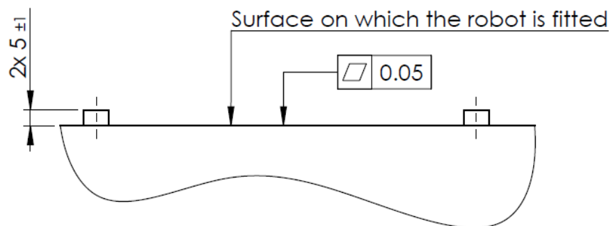
1.2: Szerelőlemez robotalaphoz
